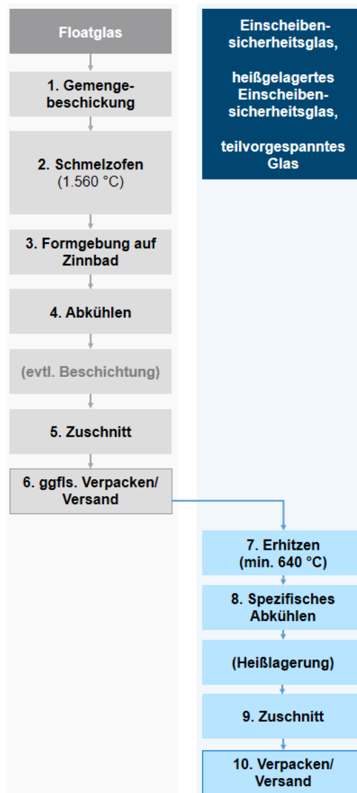
Abbildung 1 Herstellungsprozess
