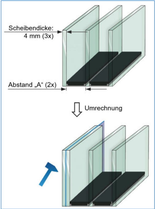
Abbildung 6 Mehrscheibenisolierverglas (© Bundesverband Flachglas e. V.)
