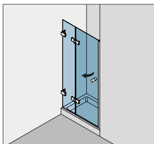
Typ(e) 200W Nischenkabine, 1 Anschlagtür am Fixteil mit Winkelbefestigung
