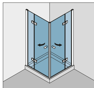
Typ(e) 220P Eckkabine, 2 Anschlagtüren an Fixteilen mit Profilbefestigung
