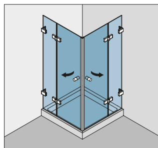
Typ(e) 220W Eckkabine, 2 Anschlagtüren an Fixteilen mit Winkelbefestigung
