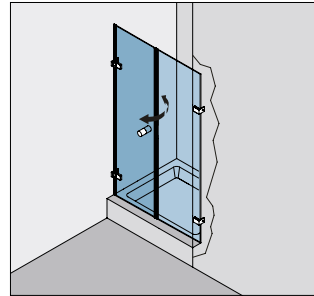
Typ(e) 110W Nischenkabine, 1 Pendeltür, 1 Fixteil mit Winkelbefestigung
