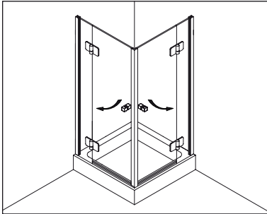
Typ / Type 220 P
