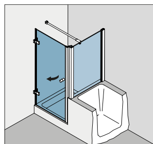
Typ(e) 131P Eckkabine an Badewanne, 1 Anschlagtür, 1 verkürzte Seiten- wand 90° mit Profilbefestigung
