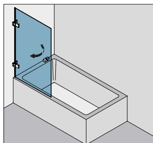
Typ(e) 170 Eckkabine, 1 Pendeltür auf Badewanne 90°
