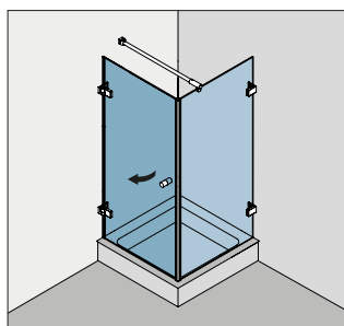
Typ(e) 130W Eckkabine, 1 Anschlagtür, 1 Seitenwand 90° mit Winkelbefestigung
